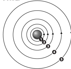
人工衛星の高度と速度の関係(円軌道)
