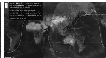
図2: 「Navstar72」の軌道は波のような形をしている。 提供: 「GoogleSatTrack」(by isana kashiwai)
