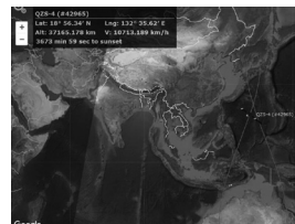
図1: 「みちびき」の軌道。 数字の8のような形をしている。
